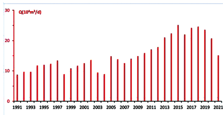
图 7 地下水开采量动态监测曲线
