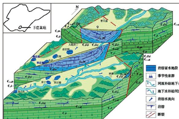
图4 羊庄盆地水文地质结构模型
