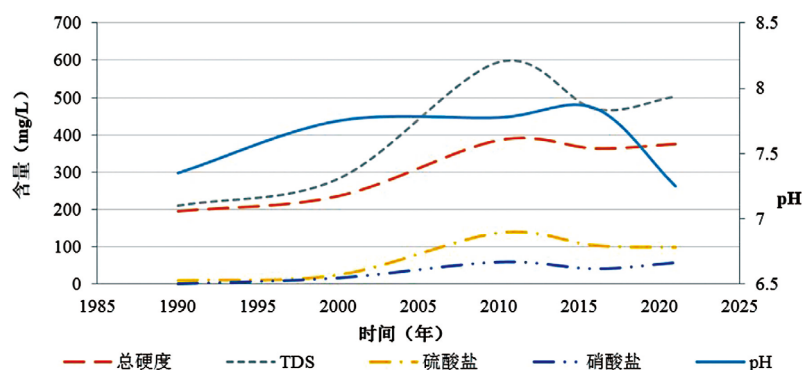
图8 水化学组分含量变化曲线
