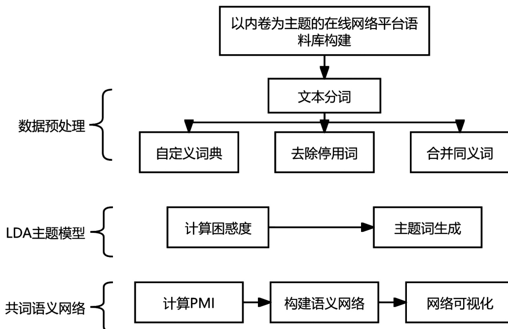
图 1 研究方法
