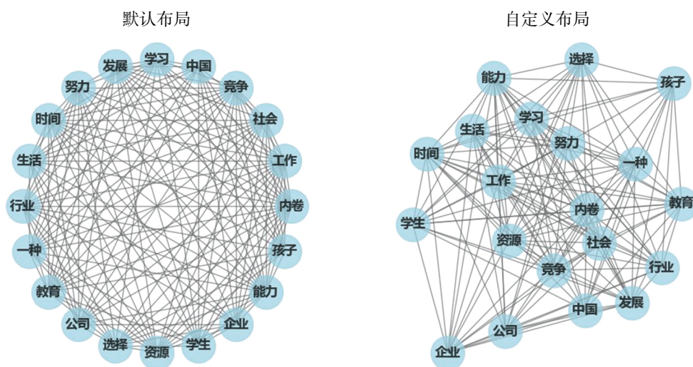
图 4 语义共现图
