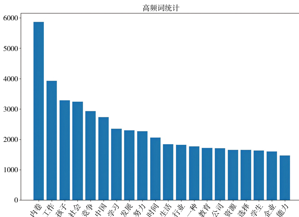
图2 词频图
